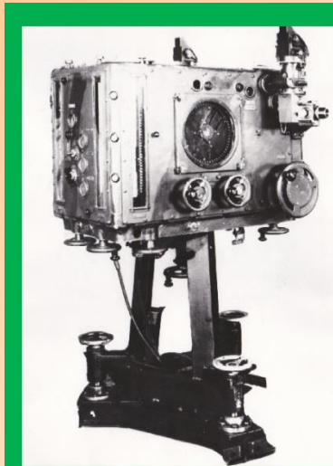
Прибор управления артиллерийск им зенитным огнем (ПУАЗО-3)
